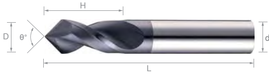
先端角度公差 \pm 0.5^\circ
