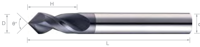
先端角度交差±0.5°
